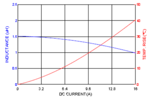
HMPL0605S-1R5
