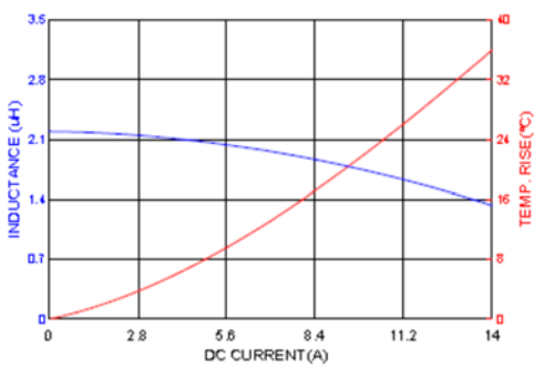
HMPL0605S-2R2
