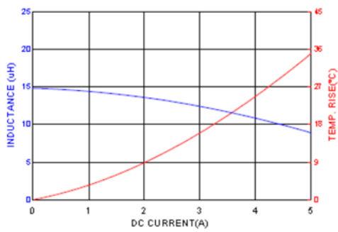
HMPL0605S-150
