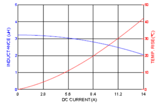
HMPL0605S-3R3
