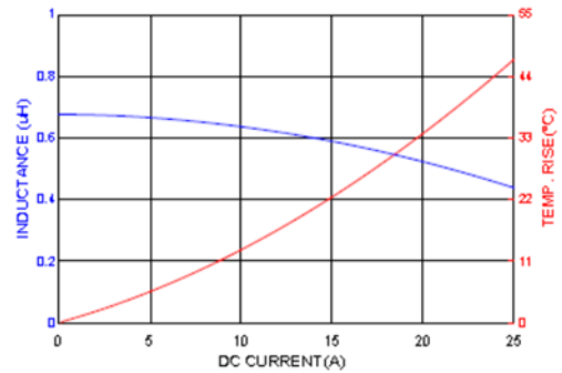
HMPL0605S-R68
