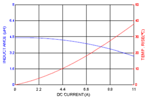
HMPL0605S-4R7
