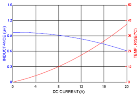
HMPL0605S-1R0
