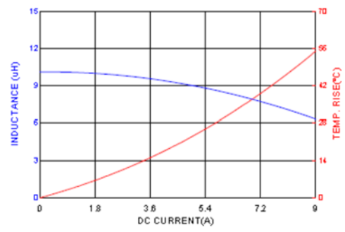
HMPL0605S-100
