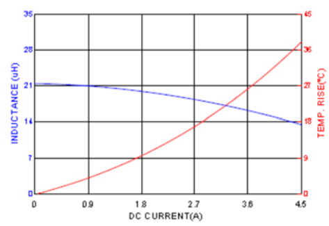
HMPL0605S-220
