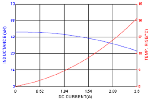
HMPL0605S-470
